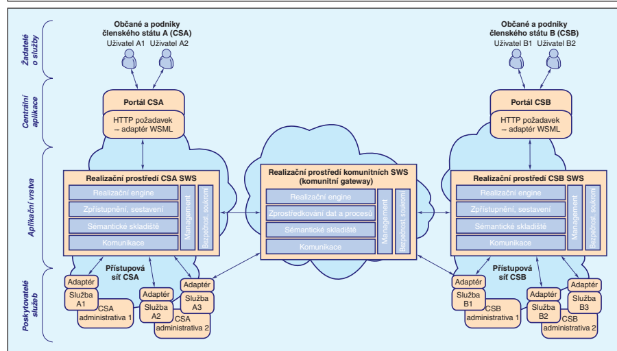
Obr. 1: Koncepce infrastruktury pro sémantické PEGS
